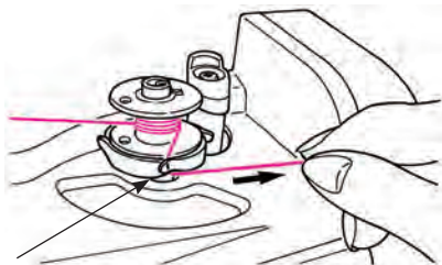
Guide (with cutter) Führung (mit Schneider) Prowadnica (z odcinaczem) направляющая (с обрезавателем)
