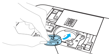
① Шпульный колпачок
