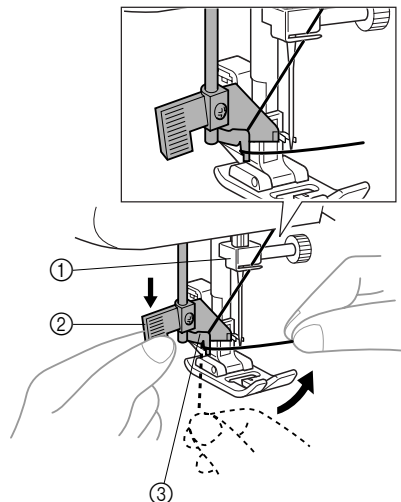
① Иголдержатель ② Рычажок устройства заправки нити в иглу ③ Направляющая
