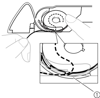
① Пружина регулировки натяжения нити
